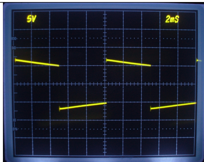
Carré 100 Hz
