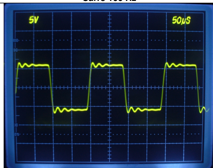
Carré 5 kHz
