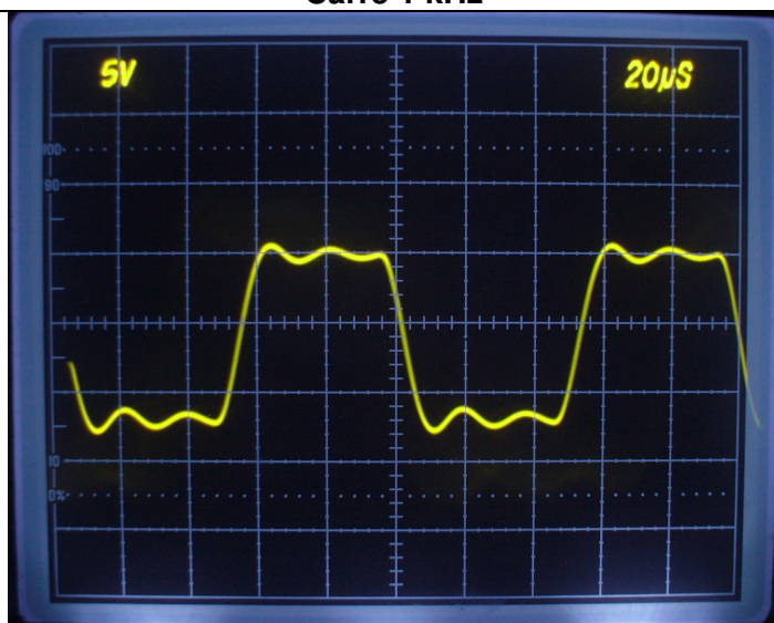
Carré 10 kHz
