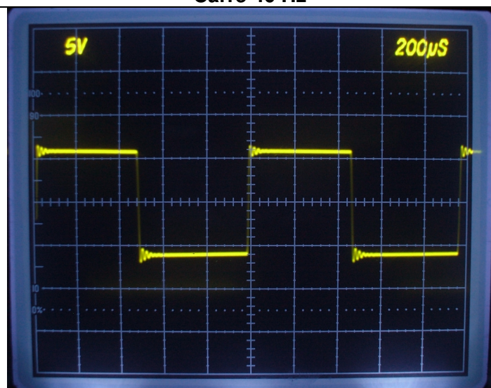
Carré 1 kHz
