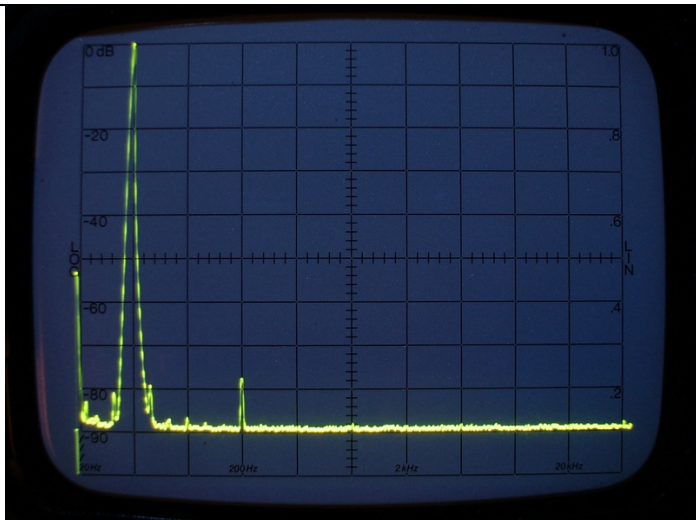
DHT à 1 kHz – 1 kHz / Div
