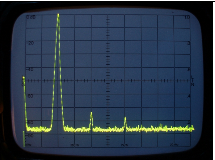
DHT à 10 kHz – 5 kHz / Div
