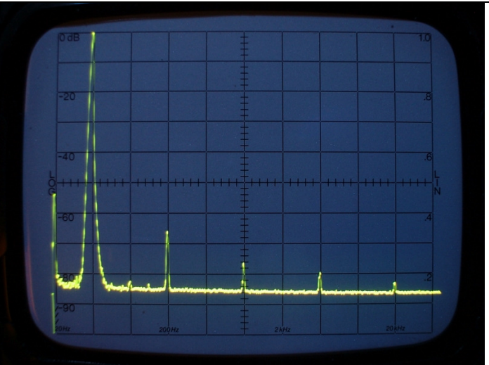
DHT à 100 Hz – 100 Hz / Div
