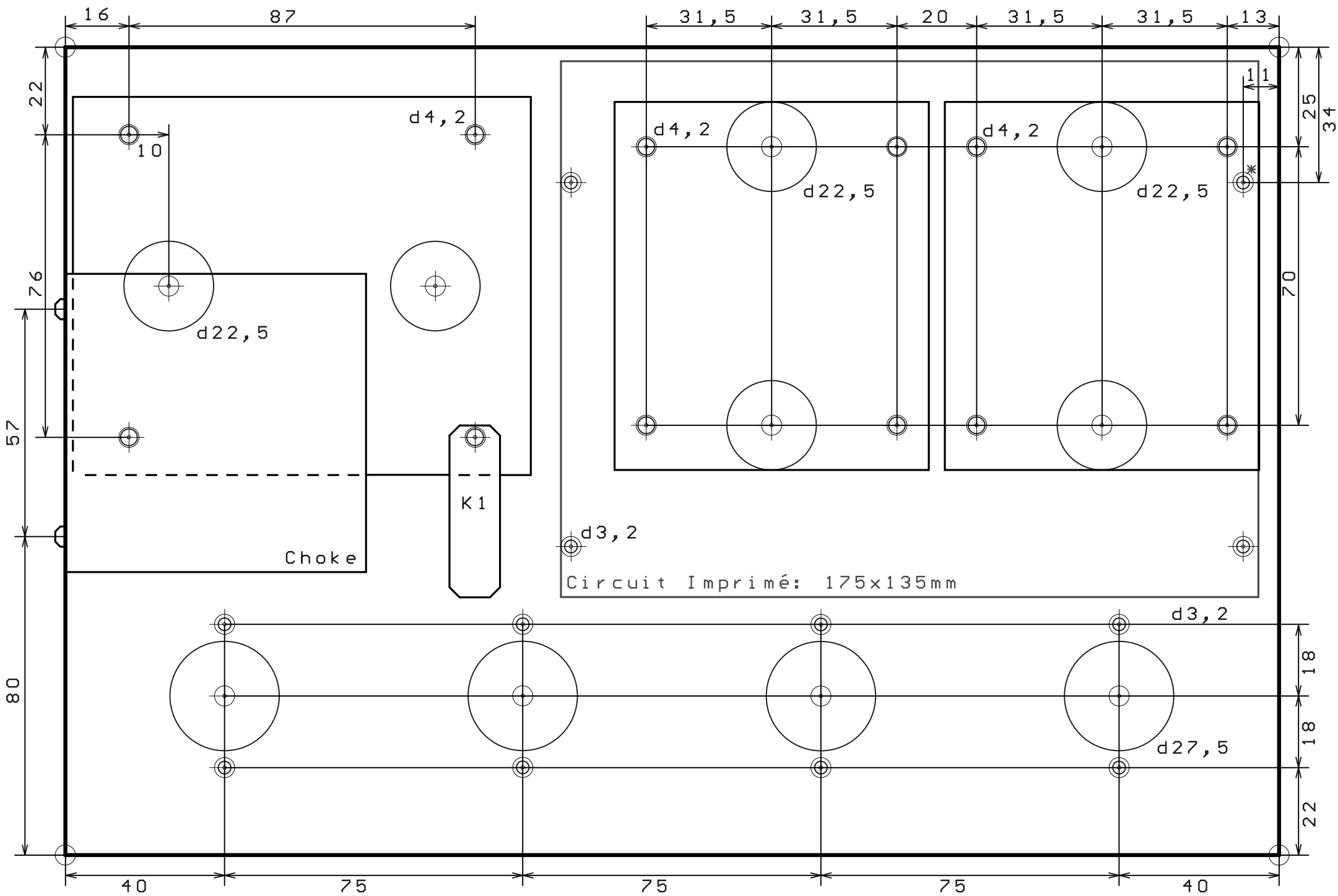
Dimensions mesurées à l'extérieur du châssis
