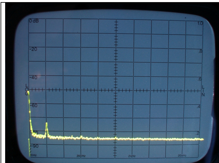
Hum & Noise - F0 → 500 Hz - Ref : 0 dBV
