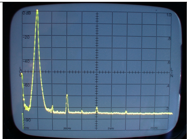
DHT à 50 Hz - F0 → 500 Hz
