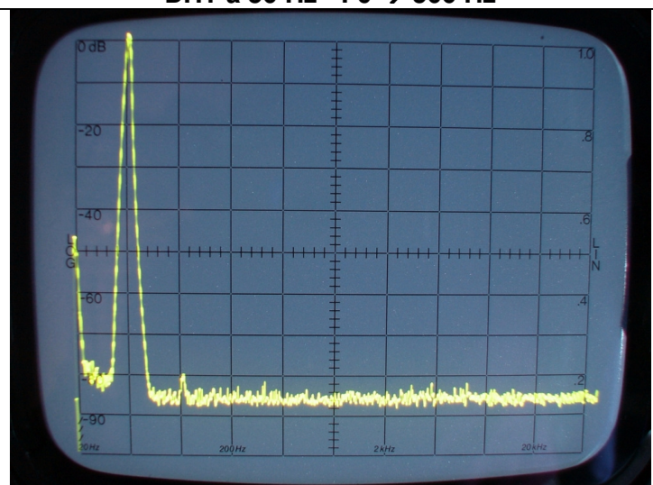
DHT à 5 kHz - F0 → 50 kHz
