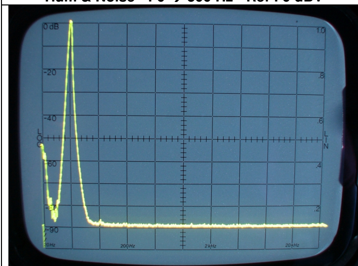
DHT à 500 Hz - F0 → 5 kHz
