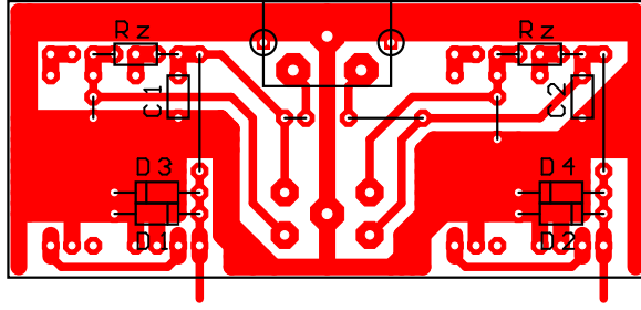
MC 1/32 Asymétrique
