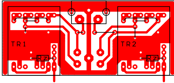
MC 1/16 Asymétrique
