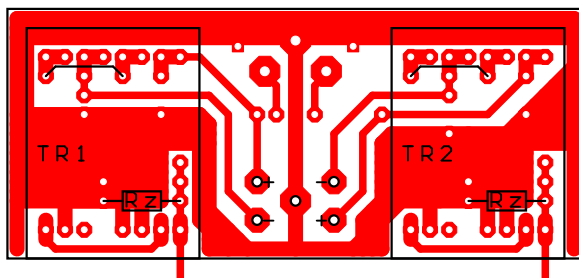
MC 1/16 Isolé
