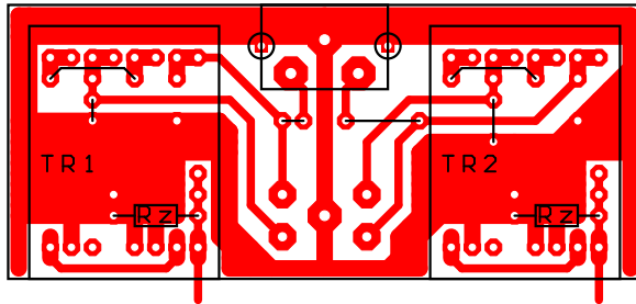
MC 1/32 Isolé
